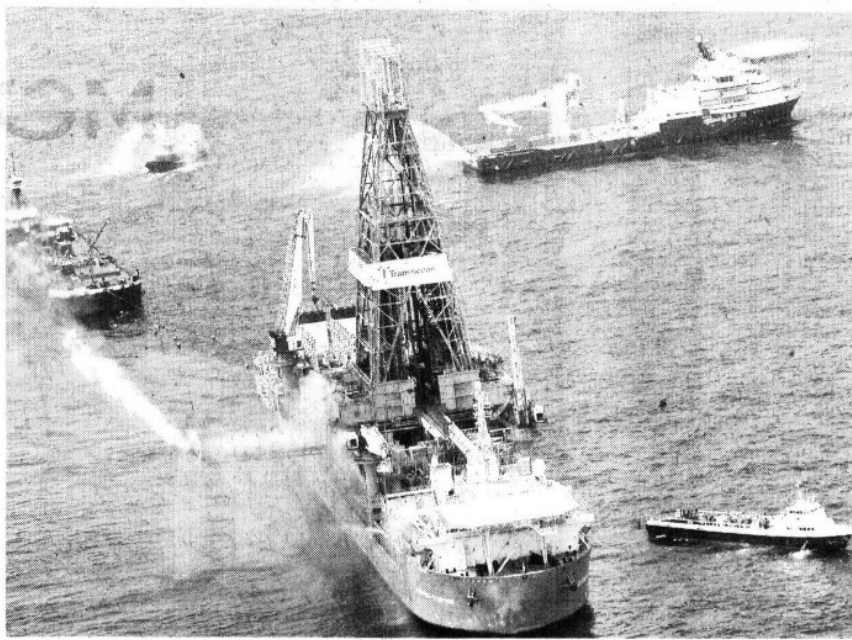
LIMPIEZA. La embarcación "Discoverer Enterprise" permanece en el sitio del derrame de petróleo y quema crudo extraído de las aguas en el golfo de México
