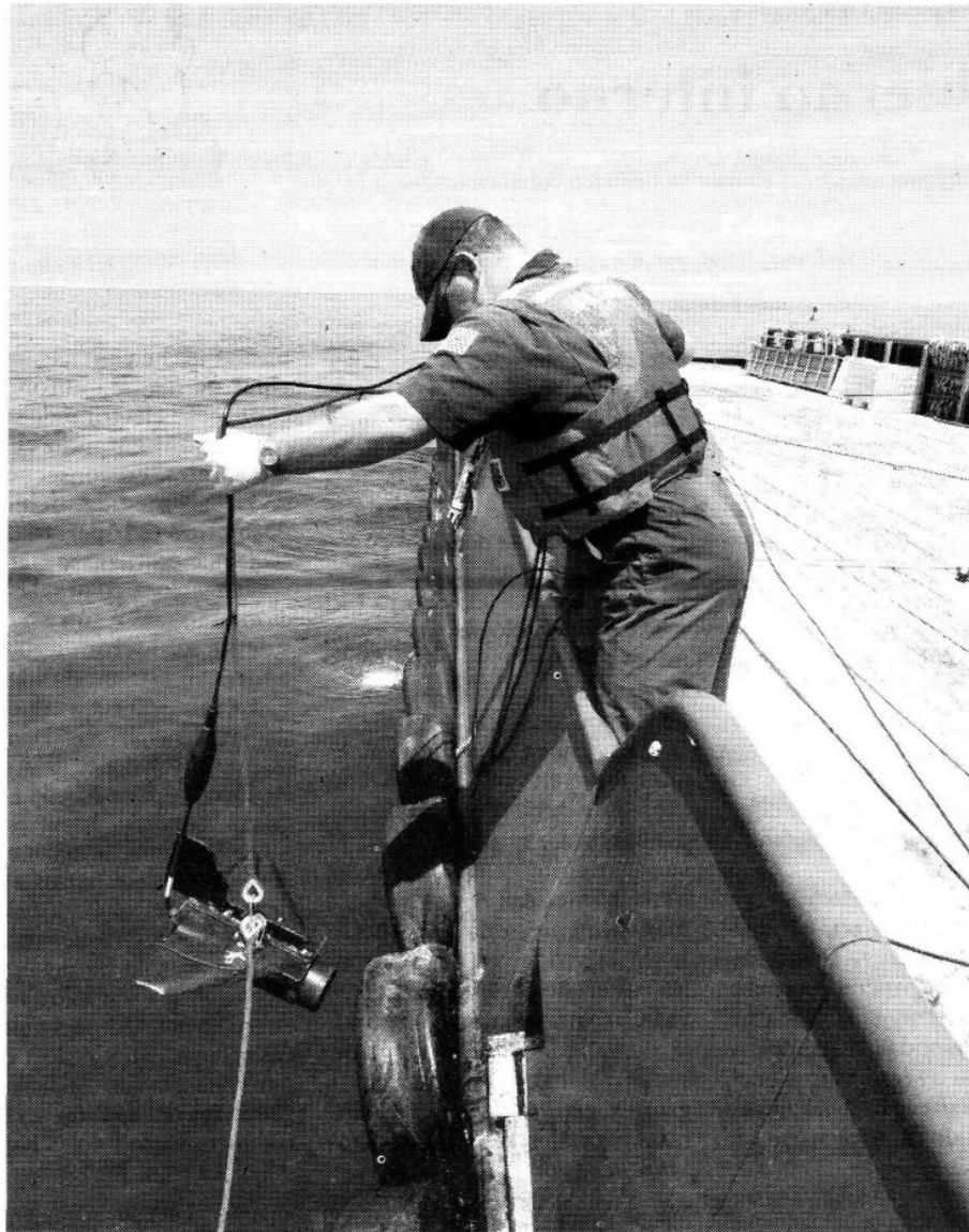
Un marino de la Guardia Costera sumerge un fluorómetro para determinar la eficacia de los dispersantes químicos. (Foto: Reuters)
